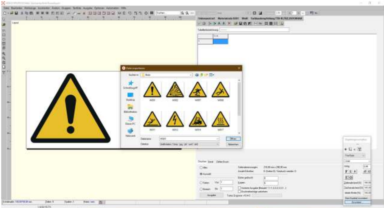
Ansicht des Schildes mit integrierter Beschriftung aus der Tabelle mit Bild aus der Symboldatei, Ausgabe an Beschriftungslaser
